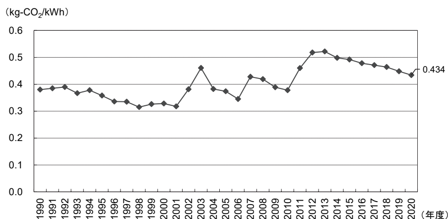
図 III-3 電力の二酸化炭素排出係数の推移
