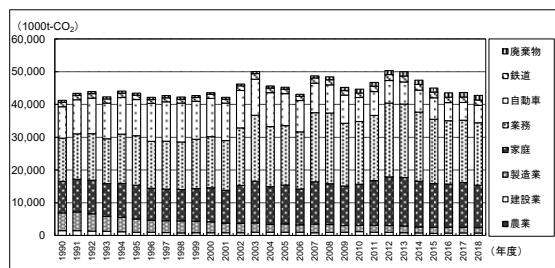
図 I-1 23 区における部門別二酸化炭素排出量の推移 (注) 二酸化炭素は温室効果ガス排出量の中で大半を占めるため、二酸化炭素排出量についての推移を掲載している。
