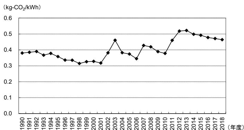
図 II-3 電力の二酸化炭素排出係数の推移
