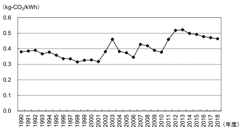
図 III-3 電力の二酸化炭素排出係数の推移
