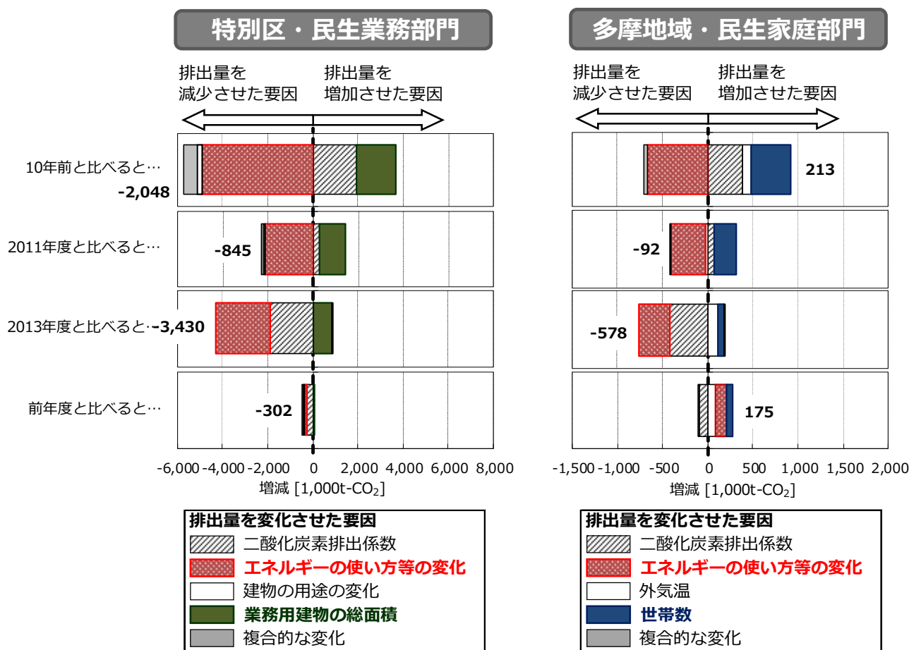
参考図 2 二酸化炭素排出量変化の要因分析 上段：10年前（2007年度）との比較／中上段：2011年度との比較 ／中下段：2013年度との比較／下段：前年度（2016年度）との比較 ※棒グラフ外に記載の数字は排出量の総変化量を示す。
