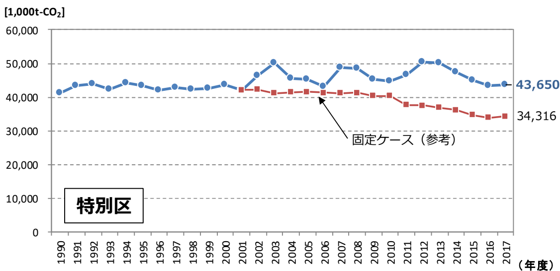
図 4.1 特別区における二酸化炭素排出量の推移
